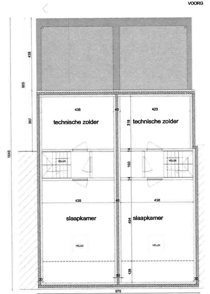
2e VERDIEPING
