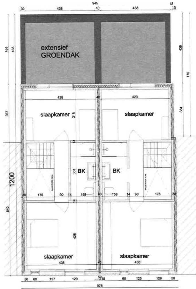
1e VERDIEPING
