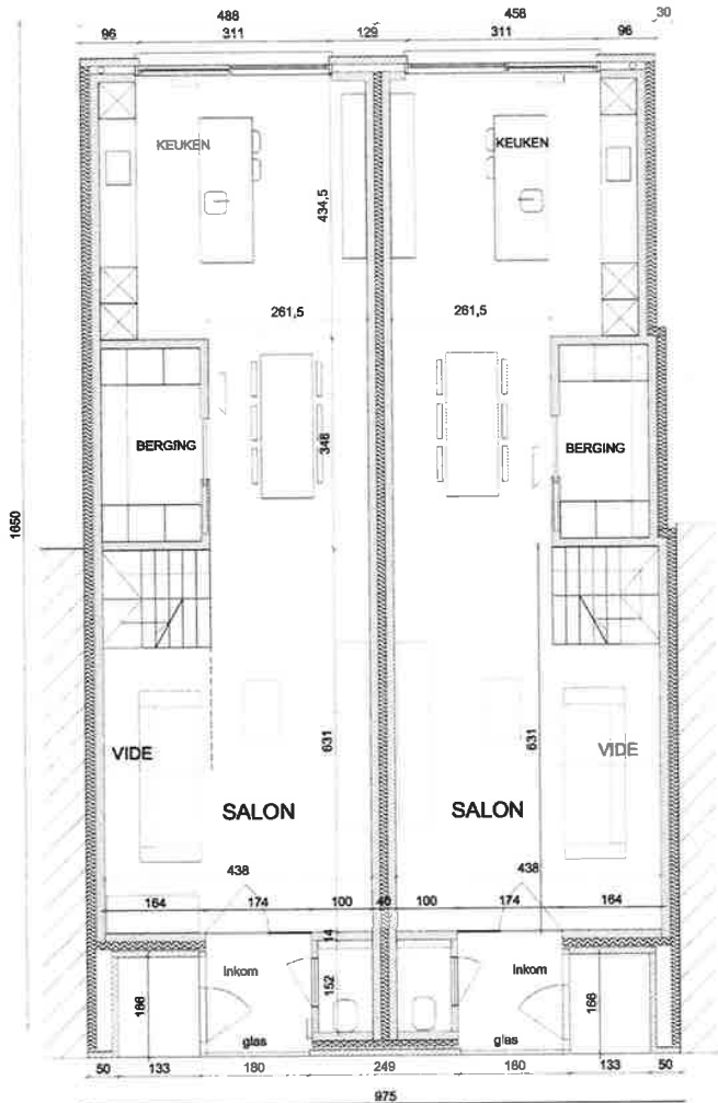
GRONDPLAN
