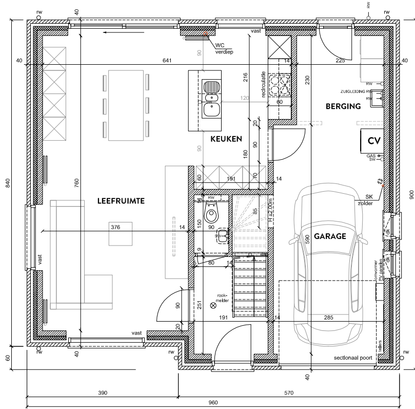
GELIJKVLOERS OPP. 84.06 M 2
